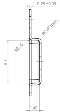
SECTION A-A SCALE 5 : 1
